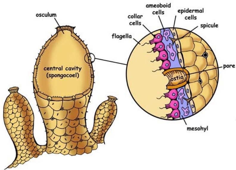
Slika 18. Građa spužve (izvor: exploringnature.org/db/view/Porifera-Sponges )
