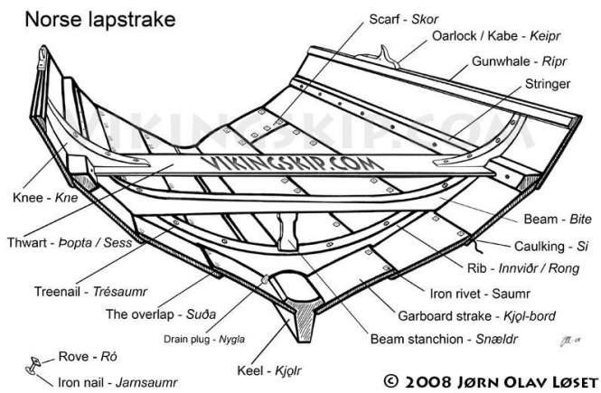
Slika 31. Dijelovi vikinške lađe
