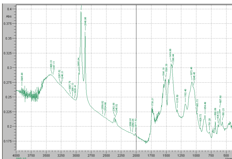
Slika 129: IR spektar uzorka crnog preslika na kosi anđela
