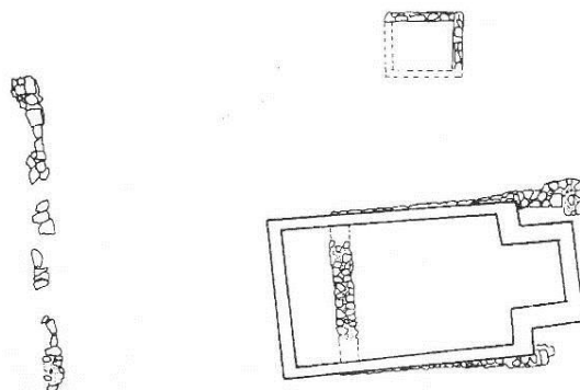
Slika 37. Tlocrt arhitektonskih ostataka iz ranijeg rimskog razdoblja (1.-3. st.)
