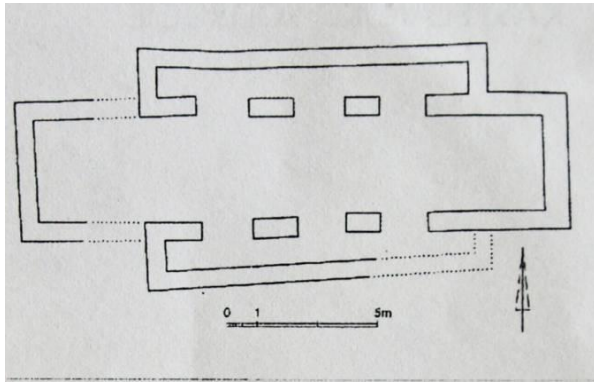
Slika 60. Tlocrt predromaničke crkve
