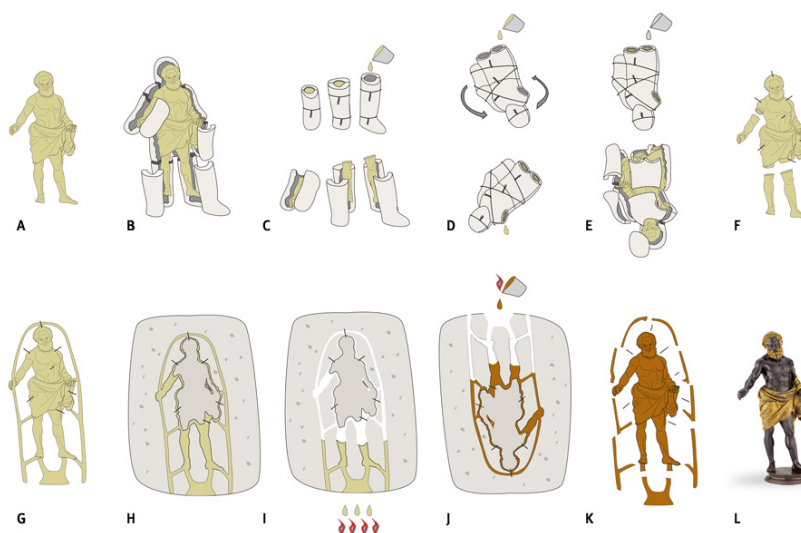
Slika 4 Proces lijevanja metodom izgubljenog voska, fotografija preuzeta sa: https://www.thesculpturepark.com/lost-wax-bronze-casting/ , pristupljeno: 25.05.2022.
